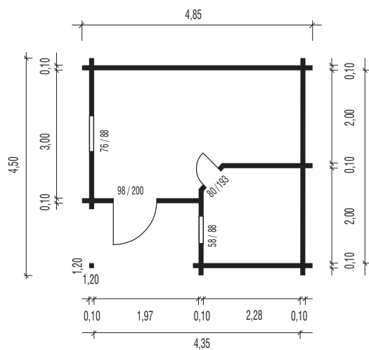
Wochenendhaus »Donau«, 80 mm Wandstärke
