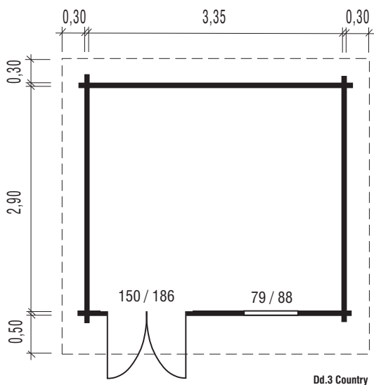
Country Dd.3 mit geraden Blenden
