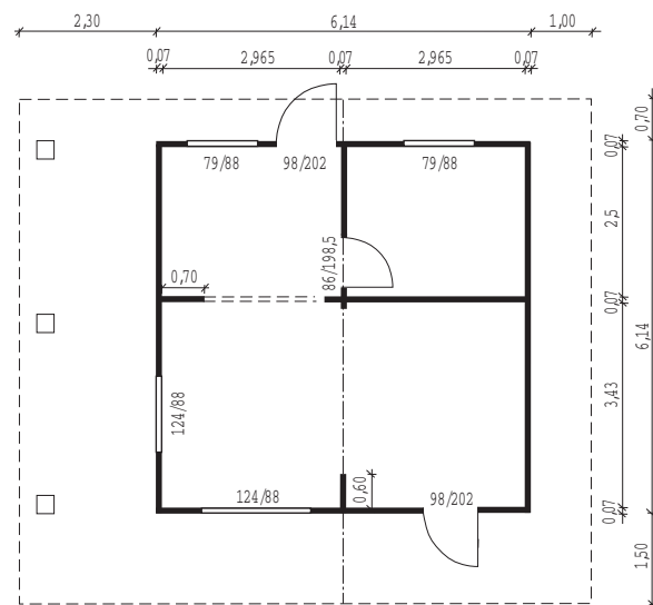
Objekt: Eisstockschießen - Vereinsheim, 70 mm Wandstärke
